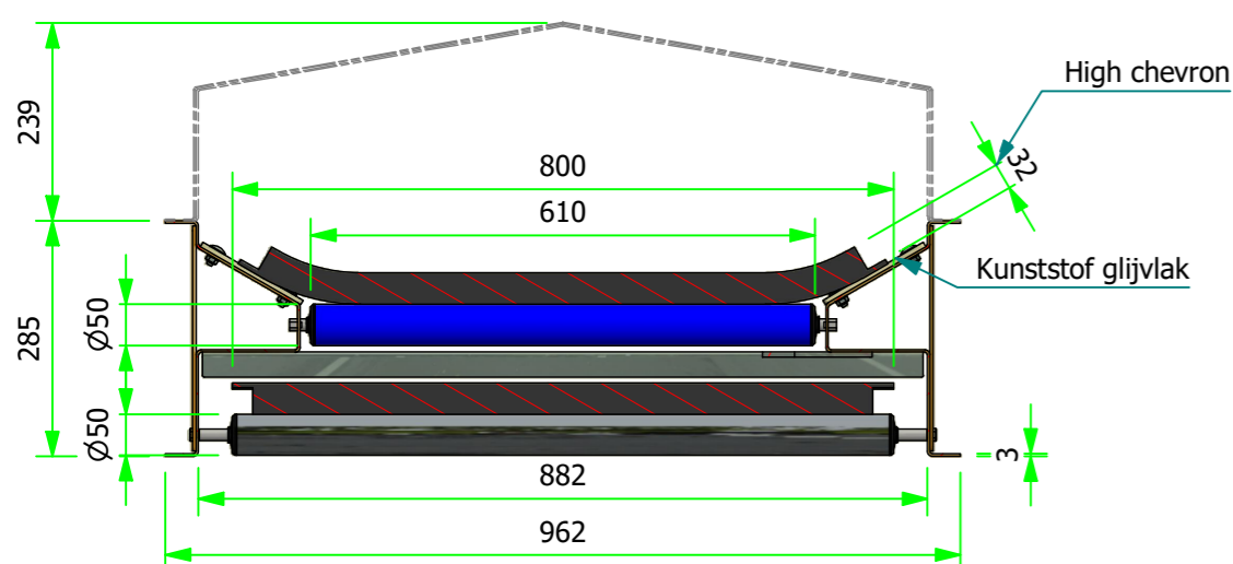
DOORSNEDE A-A ( 1 : 10 )
